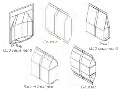
Types de sachets disponibles avec options refermables
